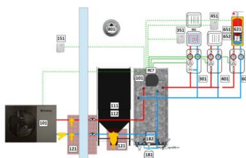
Couplage avec une chaudière granulés PERGE OptiPellet
