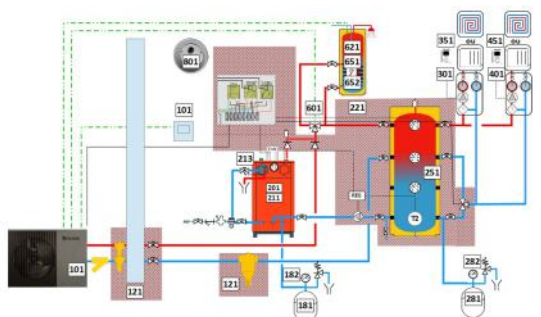
OptiPac MR290 couplée à une chaudière bois MC
