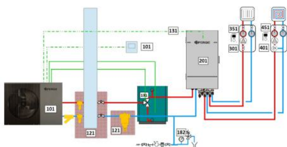
OptiPac MR290 couplée à une chaudière fioul existante
