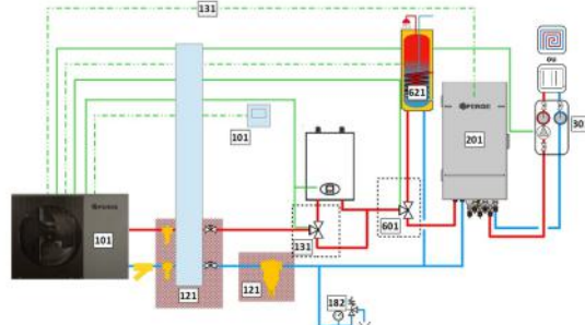
OptiPac MR290 couplée à une chaudière gaz murale existante
